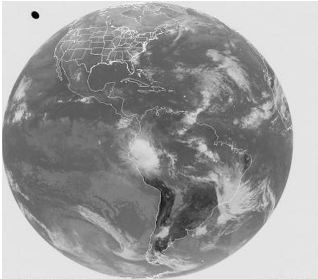
21 Nov 1999 14:45:14Z 1070 um GOES-B CIRA/NOAA-CSU
